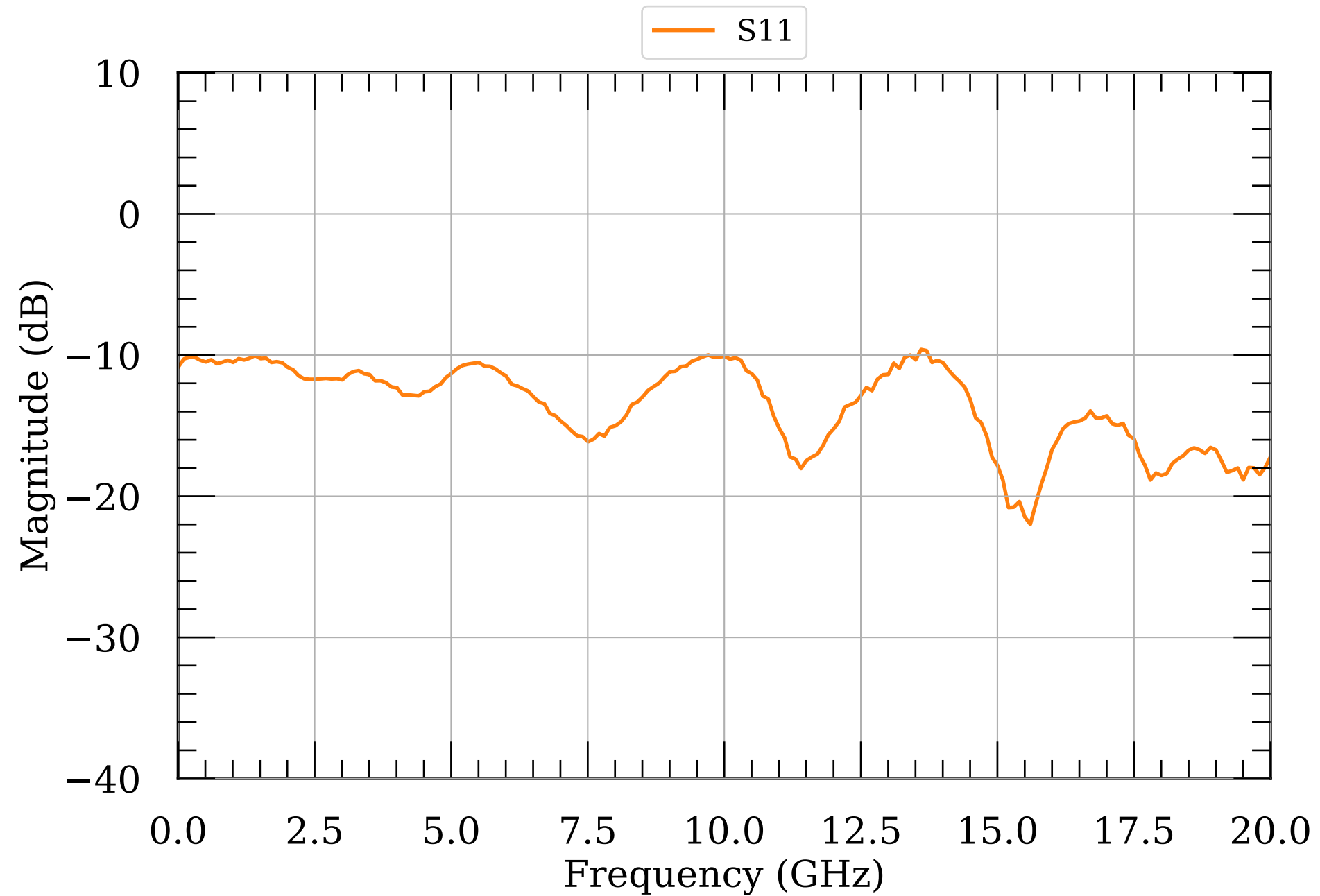
LNA S-params module024v2
